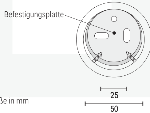
Rückansicht Wandsokkel mit Befestigungsplatte Vergrößerte Ansicht!
